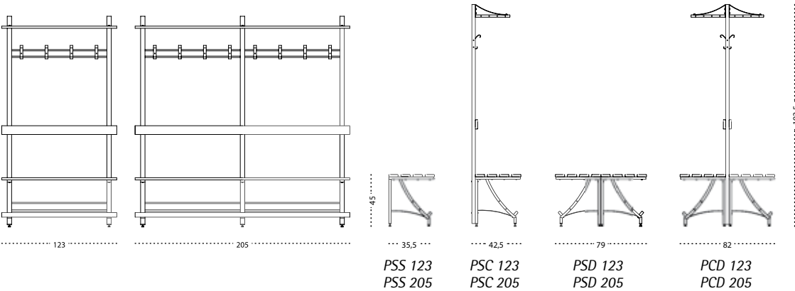
La cappelliera, alta 180 cm, è in legno e acciaio. Tutta la bulloneria è in acciaio inox.
